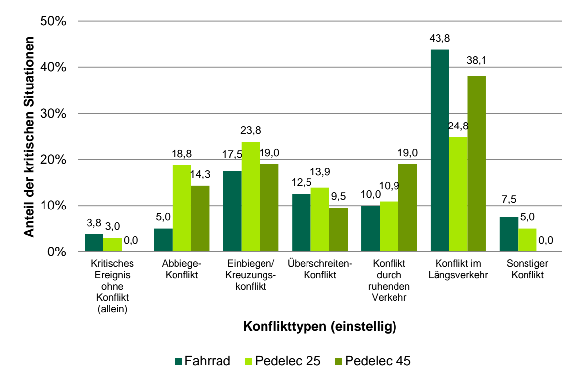
Abbildung 28: Anteil der kritischen Situationen kategorisiert nach Unfall- und Fahrzeugtyp (Daten aus kodierten Videos; gesamter Erhebungszeitraum).
