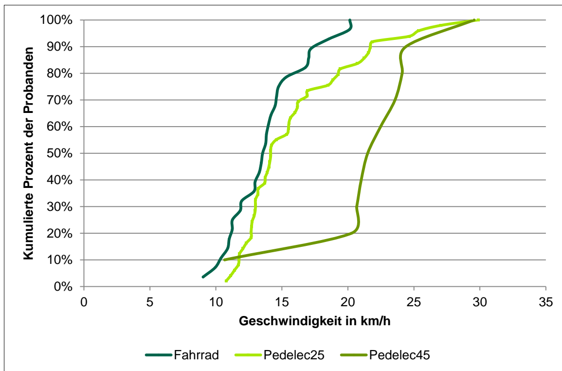
Abbildung 23: Verteilung der durchschnittlichen Geschwindigkeiten mit Standzeiten nach Fahrzeuggruppen (Radsensordaten; gesamter Erhebungszeitraum; Fahrrad: n = 28 ; Pedelec25: n = 49 ; Pedelec45: n = 10 ).
