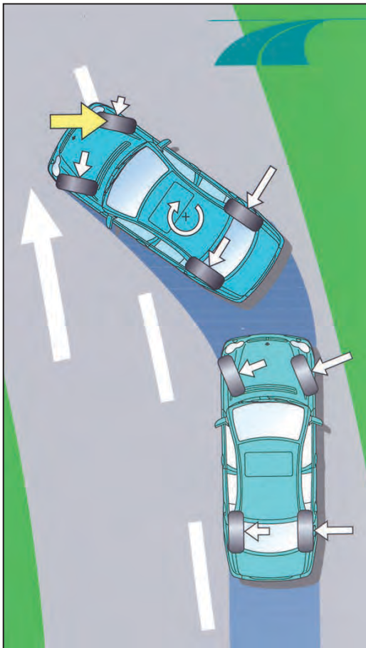
Abbildung 1: Übersteuern - das Heck bricht aus; Fahrzeugstabilisierung durch automatischen Bremseneingriff am rechten Vorderrad (Quelle: Mercedes-Benz)
