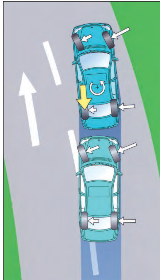
Abbildung 2: Untersteuern - die Vorderräder schieben nach außen; Fahrzeugstabilisierung durch automatischen Bremseneingriff am linken Hinterrad (Quelle: Mercedes-Benz)
